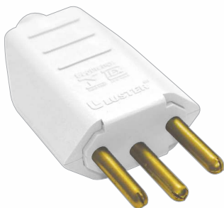
Plugue Macho 2P+T - BCO 10 A / 250 V~
